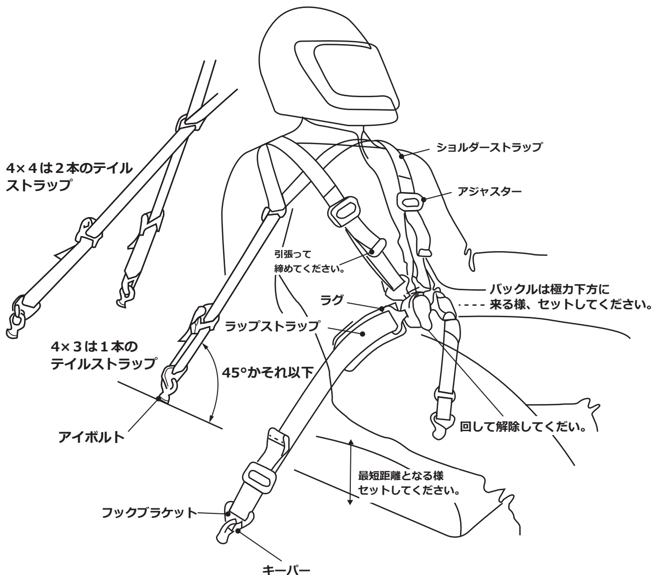
Fig 1- 全体構成図 -CLUB4
