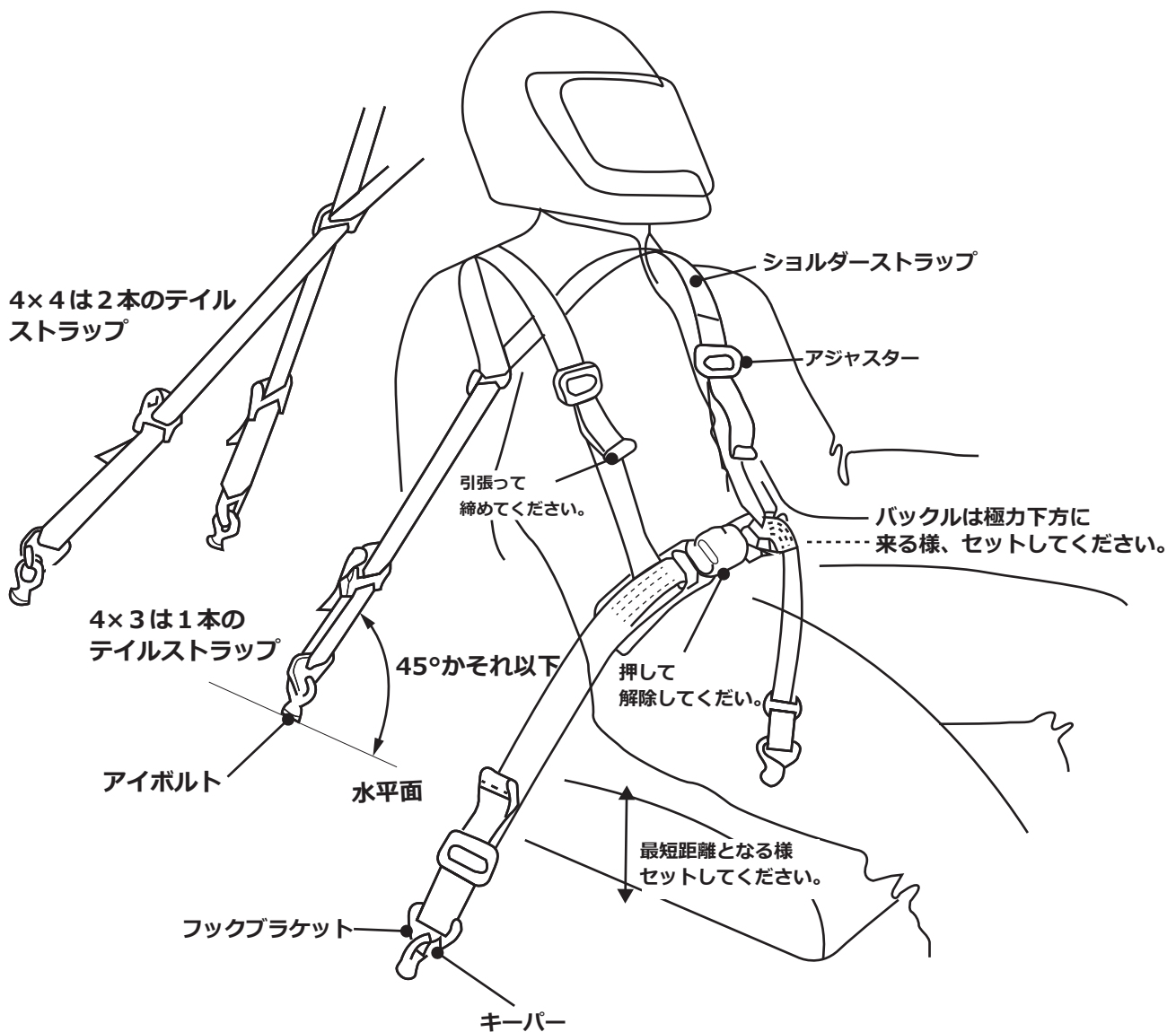
Fig 1- 全体構成図 -Supersports
