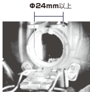
(図2) ヘッドライト側口金必要寸
